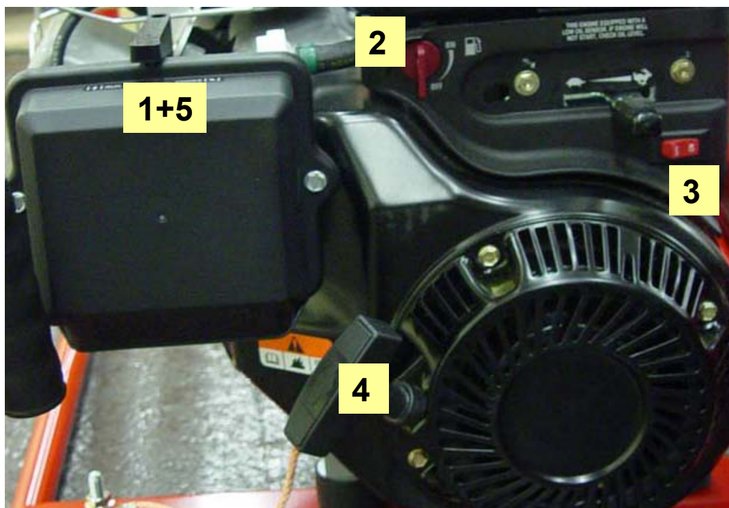
Рис. 4.2: Пуск мотора
